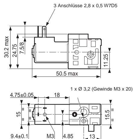
Zwischenbaustein 81 547 5
