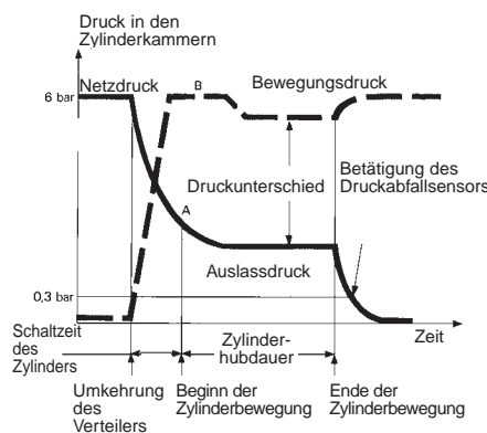
Druckaufbau in den Kammern eines doppelt wirkenden Zylinders
