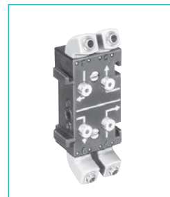
81 552 601 Abzweigungsplatte
