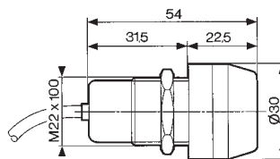
84 150 201 - 84 150 202 84 150 203 - 84 150 204
