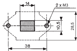
Vierkanthebel
