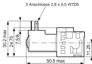
Anfangs-/Endplattensatz (1 Paar) 81 547 0
