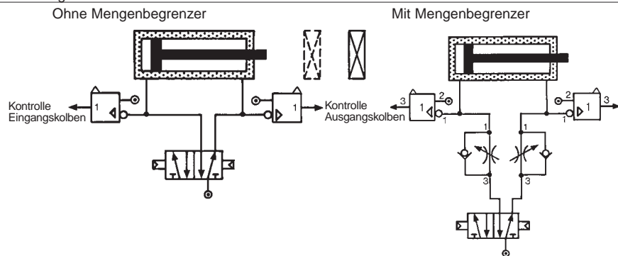
Druckaufbau in den Kammern eines doppelt wirkenden Zylinders
