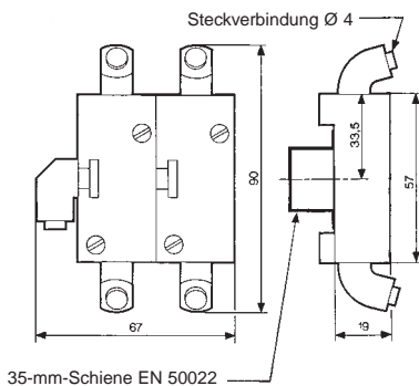
81 542 002 (zur Erinnerung 81 523 201/601)
