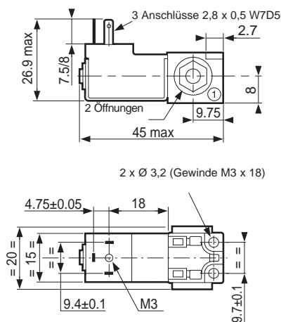
Einzelgrundplatte 81 546 0
